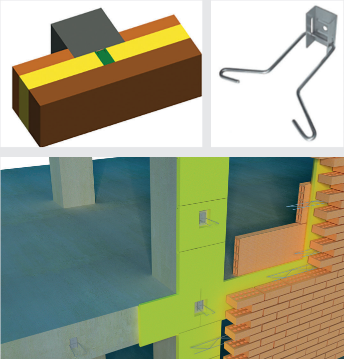
PT12. Anclaje puntual
