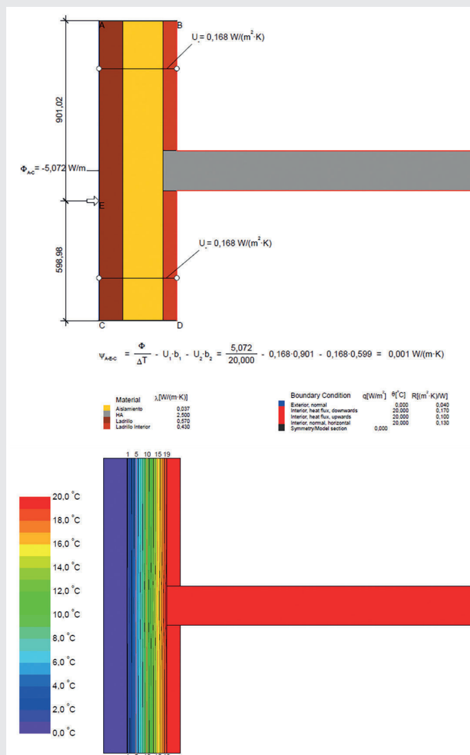
Figura 7: Ejemplo cálculo detallado de puente térmico. Encuentro de la fachada Structura con el frente del forjado. PT03 ME – EQ-20 200 MM. Cálculo detallado e isotermas.
