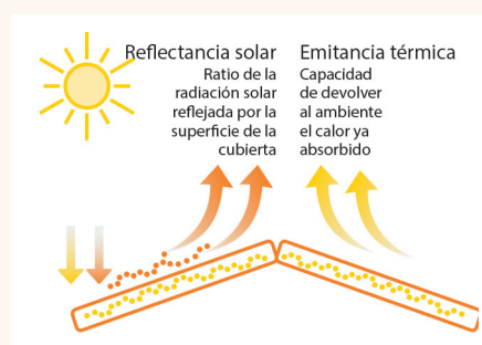
Figura 11. Reflectancia y emitancia de una cubierta inclinada.
