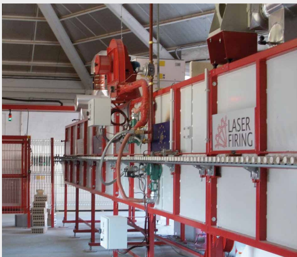
Foto 3 Horno con detalle de los dos equipos láser
