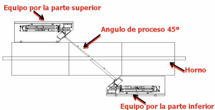
Figura 3.- Integración láser
