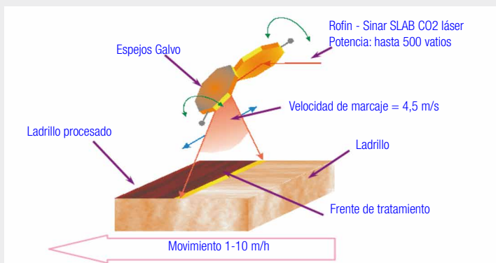
Figura 1.- Proceso de tratamiento
