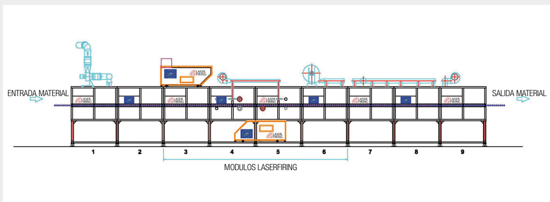
Figura 2.- Horno Laserfiring
