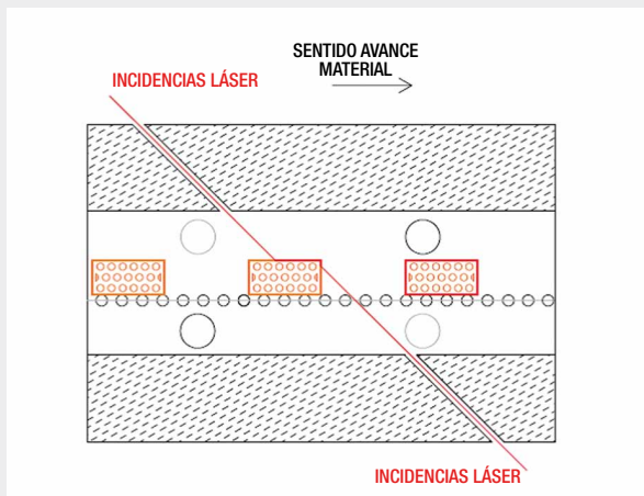
Figura 4.- Incidencia del láser en las piezas cerámicas
